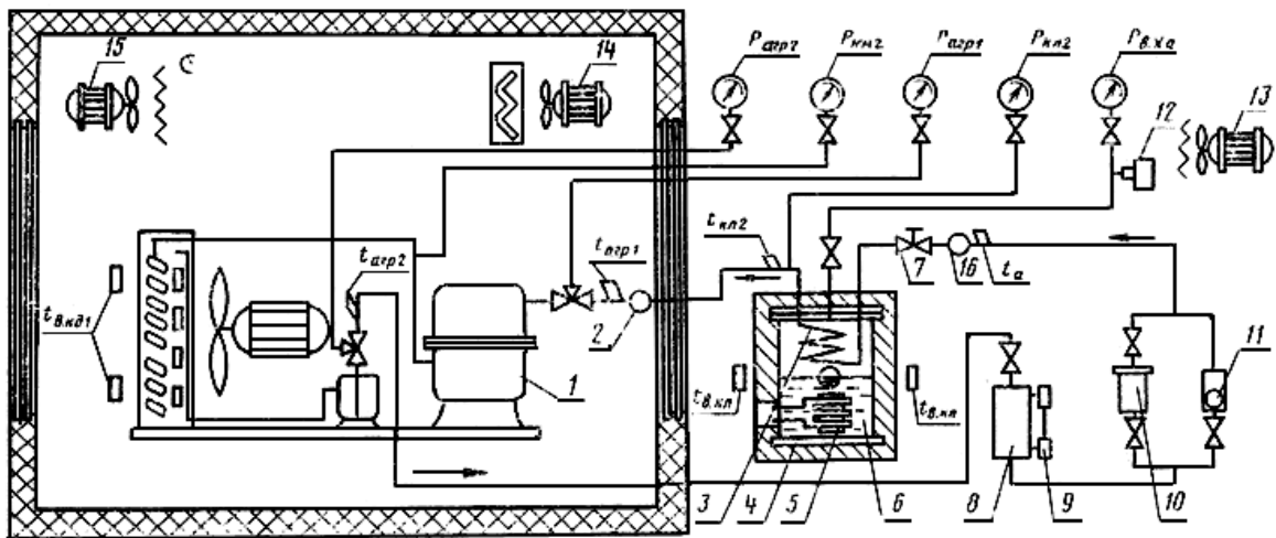
Схема стенда с электрическим калориметром
