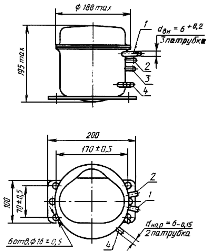
1 - нагнетательный патрубок; 2 - операционный патрубок; 3 - всасывающий патрубок; 4 - патрубки устройства для дополнительного охлаждения Черт. 1
