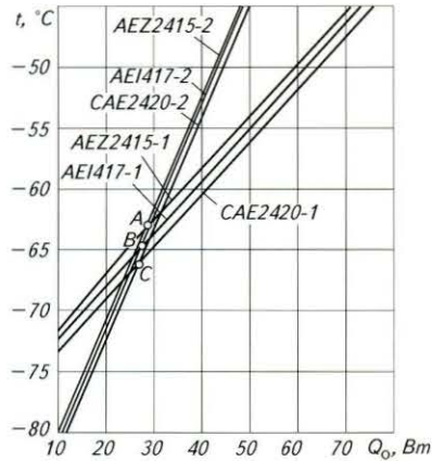
Рис. 4. Сводный график зависимости температуры в камере термостатирования от тепловой нагрузки
