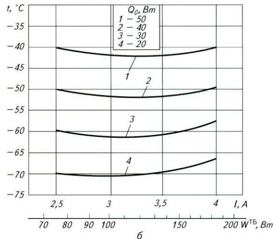
Рис. 3. Зависимость температуры в камере от силы тока питания термобатарей при различных тепловых нагрузках:
